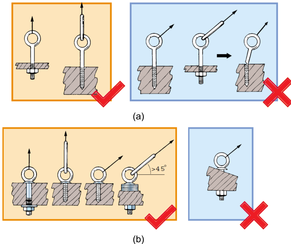
Rajah 7.7 Kaedah yang betul dan salah untuk ikatan (a) bol-tindik tidak berkolar dan (b) bol tindik berkolar ( Occupational Safety & Health Council, Hong Kong, 2002 )
