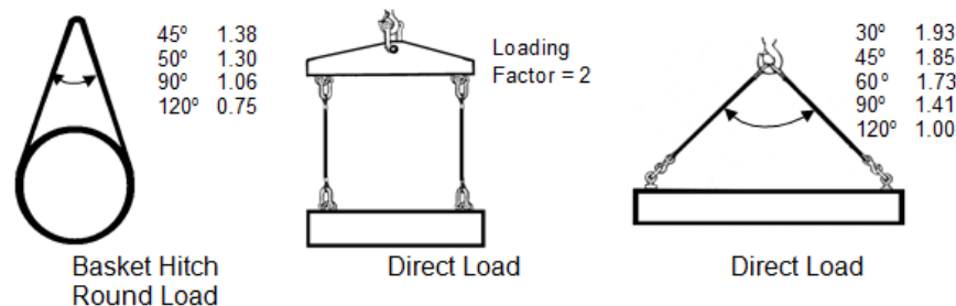
Rajah 5.8 Faktor beban dengan pelbagai kaedah ikatan anduh serta beban yang berbeza bentuk. (www.cranecrew.com)
